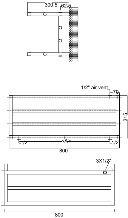
SMART U welded/sudat (for RAL / pentru vopsit)
