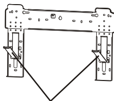
Desfaceți suportul de pe placa de montare
